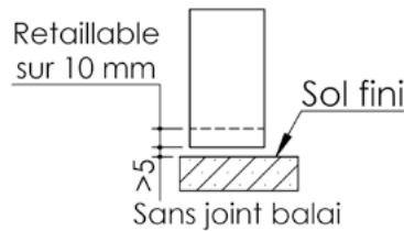
Variante bas de porte
