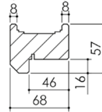
Huisserie isophonique
