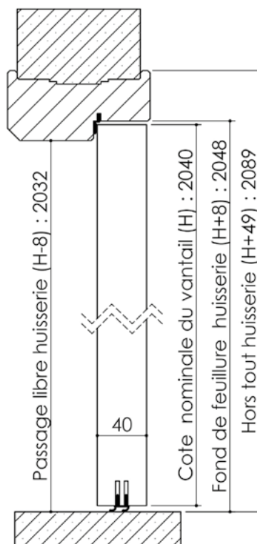
Huisserie isophonique
