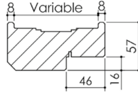
Huisserie isophonique Variable
