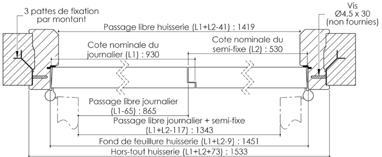
Seuil à la suisse + joint balai
