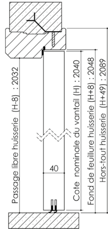
Huisserie isophonique Variable
