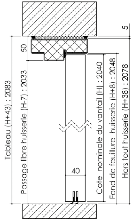
Huisserie isophonique
