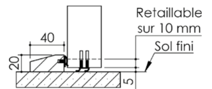
Seuil à la suisse + joint balai
