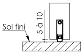
Plinthe automatique
