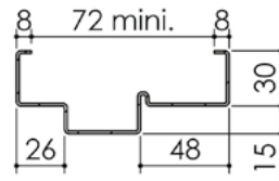
Huisserie isophonique
