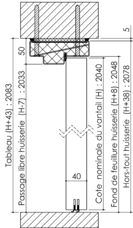
Huisserie isophonique
