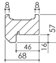
Huisserie isophonique
