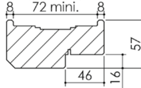
Huisserie isophonique
