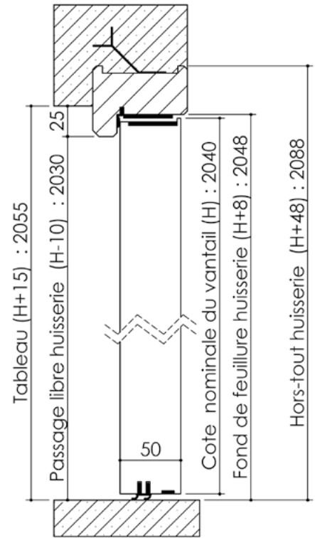
Détail de feuillure centrale
