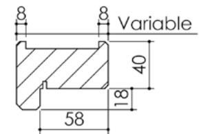
Huisserie isophonique
