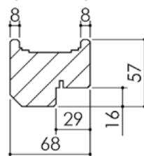
Huisserie isophonique
