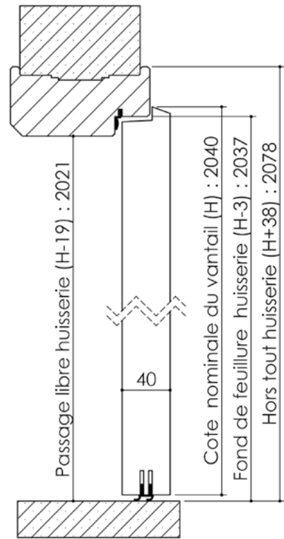
Huisserie isophonique
