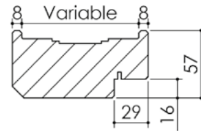
Huisserie isophonique
