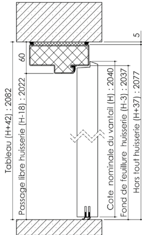
Huisserie isophonique
