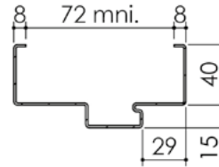
Huisserie isophonique
