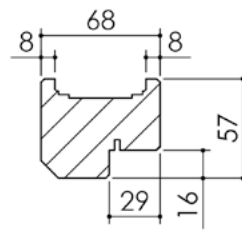
Huisserie isophonique
