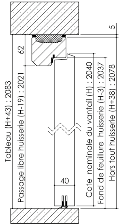
Huisserie isophonique
