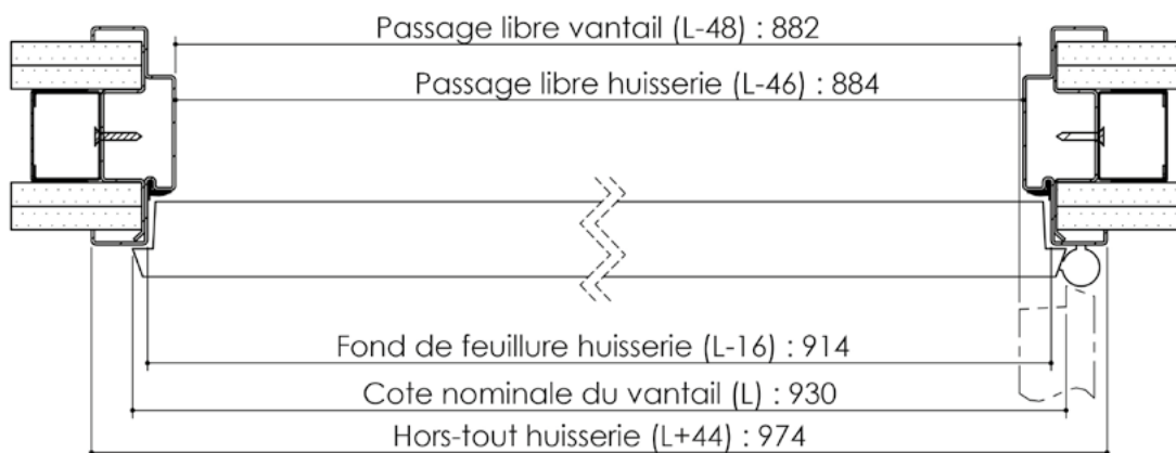
Seuil à la suisse + joint balai
