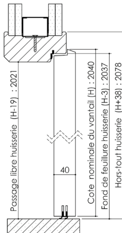
Huisserie isophonique
