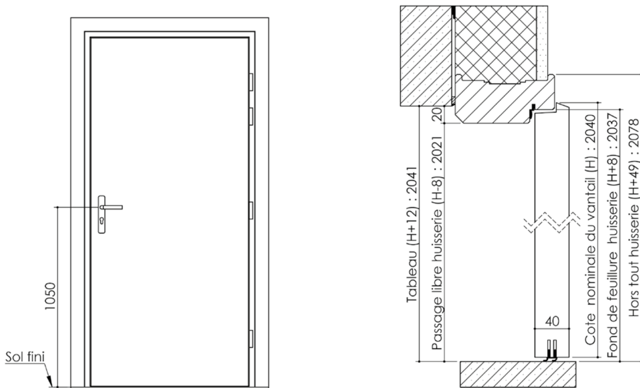
Huisserie isophonique
