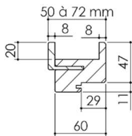
Huisserie isophonique
