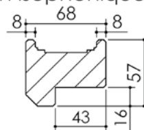
Huisserie non isophonique
