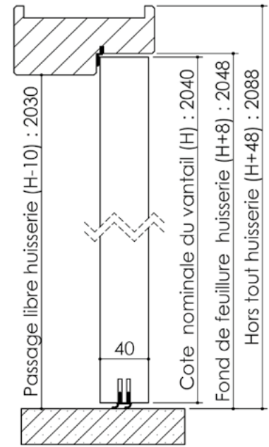
Huisserie isophonique
