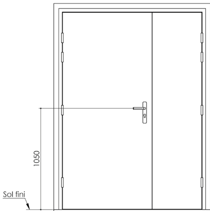
Variante d'étanchéité
