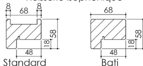
Huissierie isophonique
