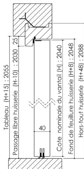
Huissierie isophonique
