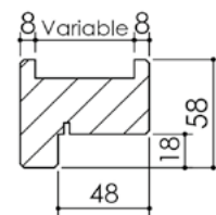
Huisserie isophonique
