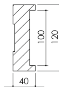
Montant côté battement en configuration 1 vantail
