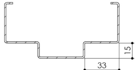
Huisserie non isophonique Pavillon 31, 31 CR3
