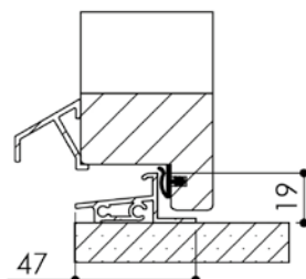
Seuil alu PMR Version Résidence C Metalforce Coursive BP1
