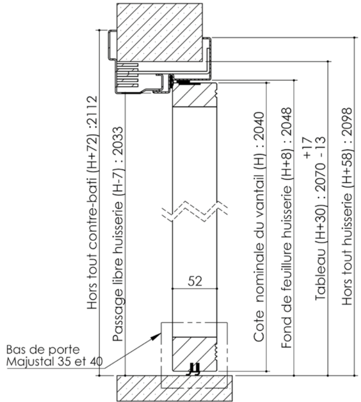
Huisserie isophonique
