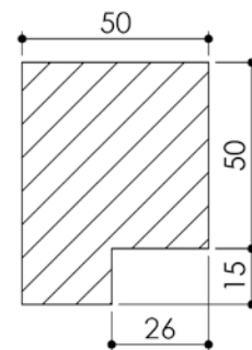
Huisserie non isophonique
