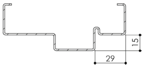
Huisserie isophonique
