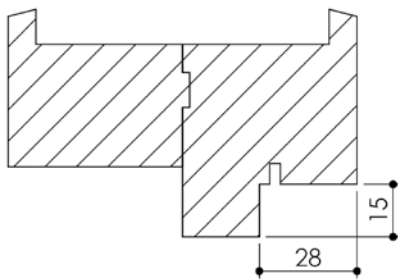
Huisserie isophonique
