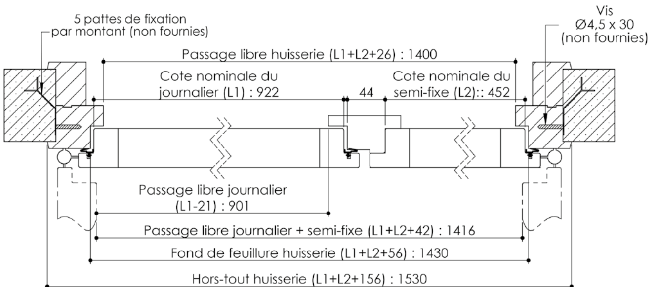
Huisserie isophonique
