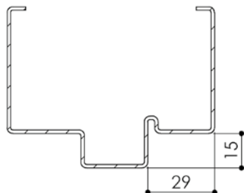
Huisserie isophonique
