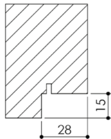
Huisserie isophonique
