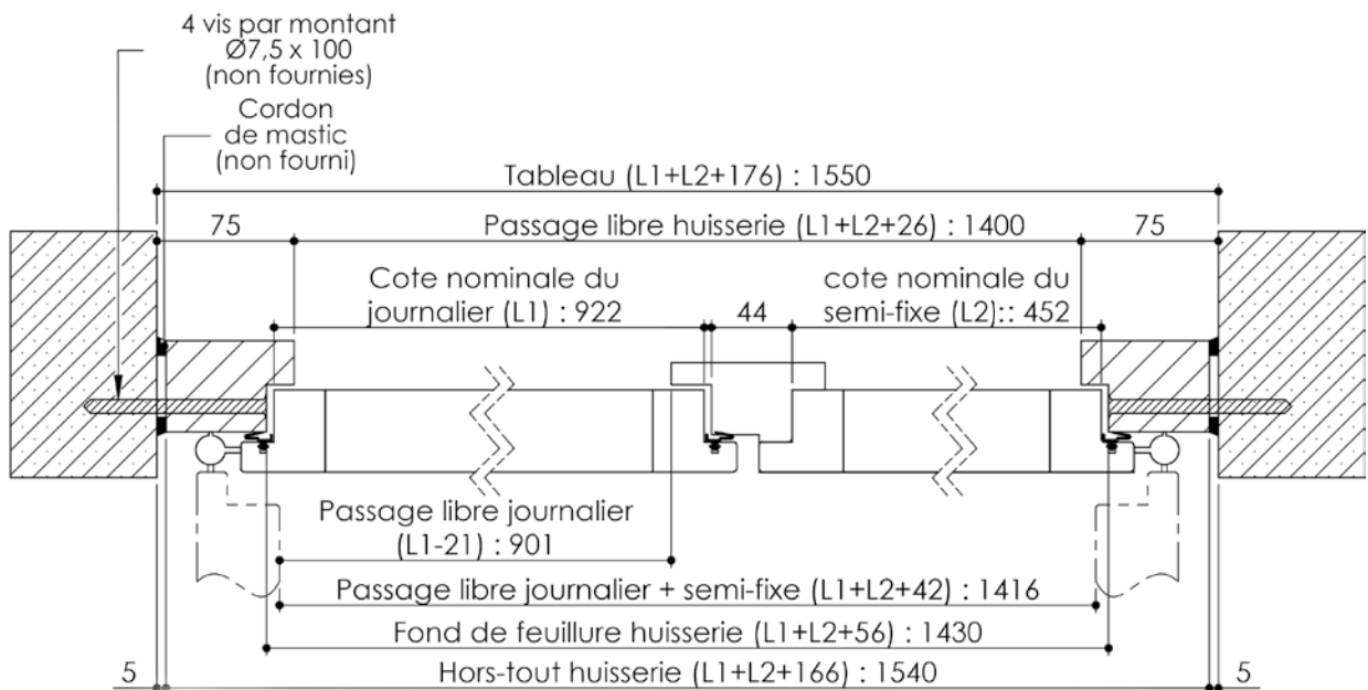
Huisserie isophonique
