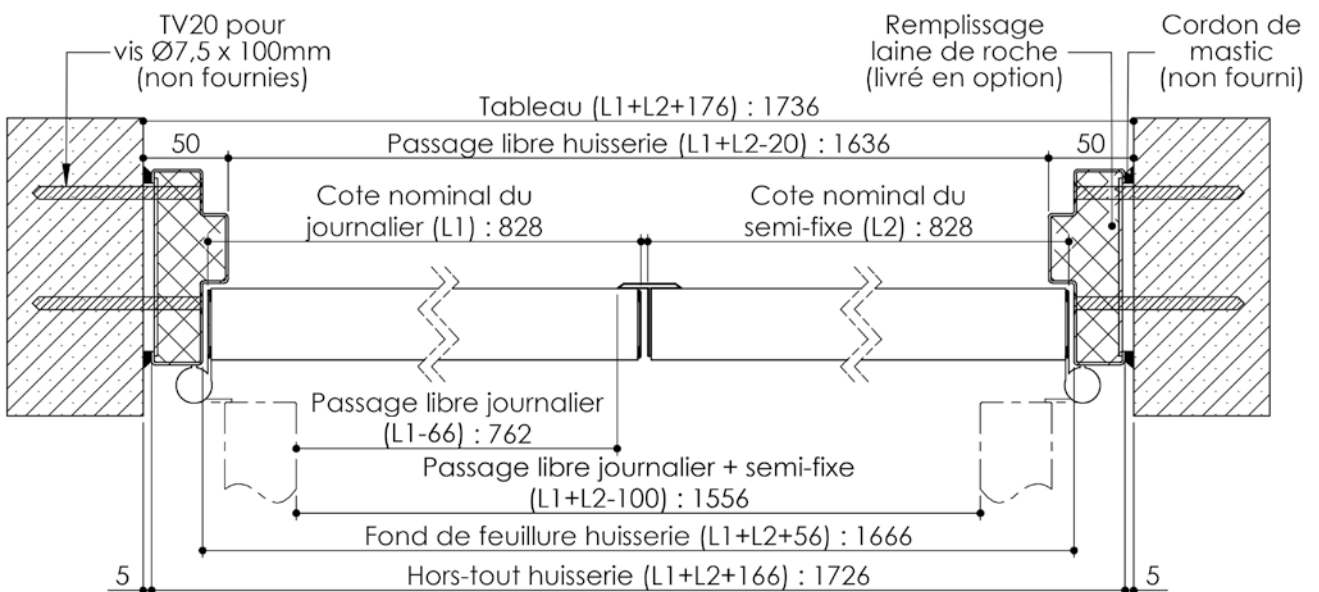
Huisserie isophonique
