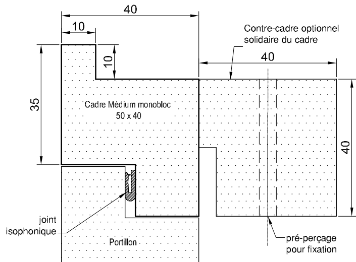
Coupe de principe modèle MM30-35C
