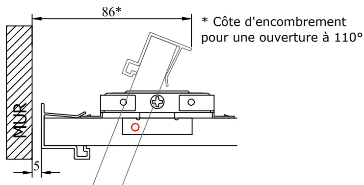
Tirant Droite
