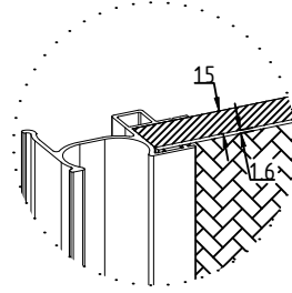
Leguan : épaisseur 1.6 mm Panneau : épaisseur 15 mm Hauteur Total maxi : 2600 mm
