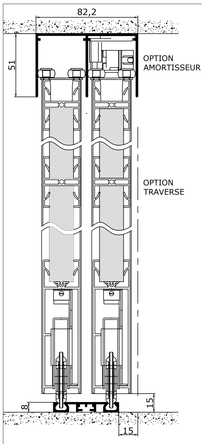
VUE EN COUPE
