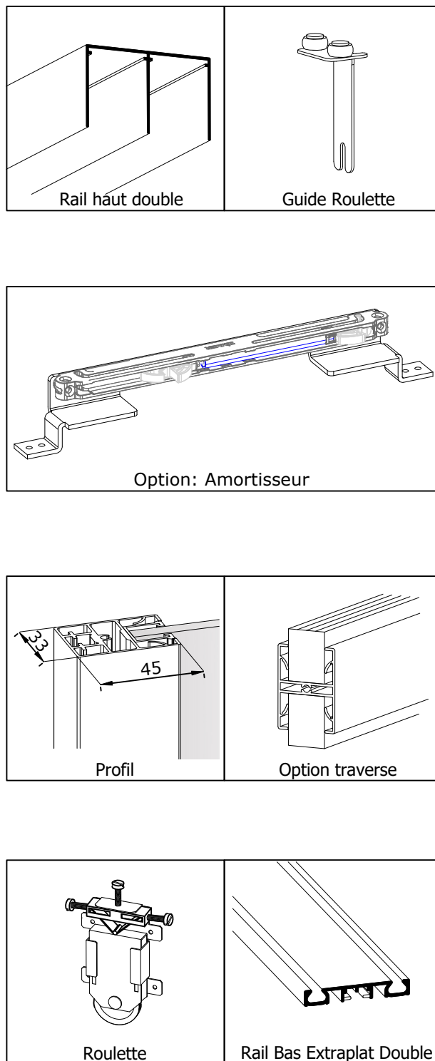
VUE DES ÉLÉMENTS
